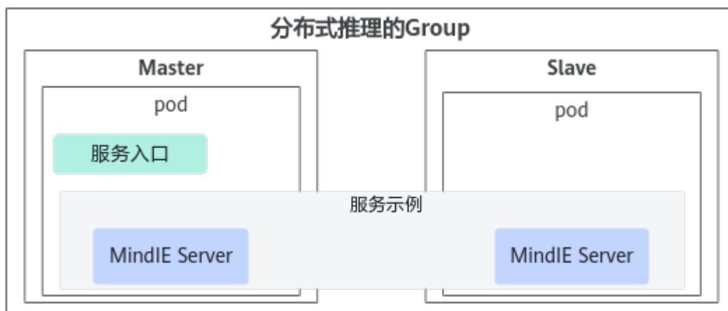
图 3-14 分布式多机场景部署架构图
