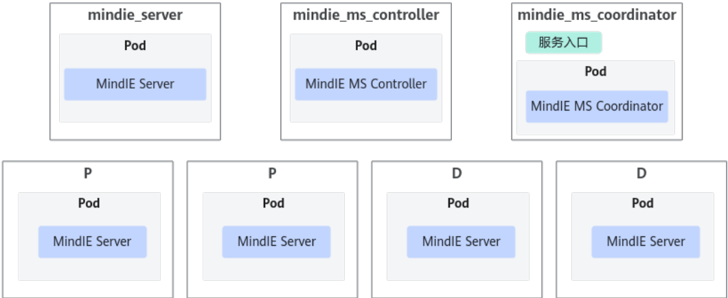
图 3-16 PD 分离的部署形态
