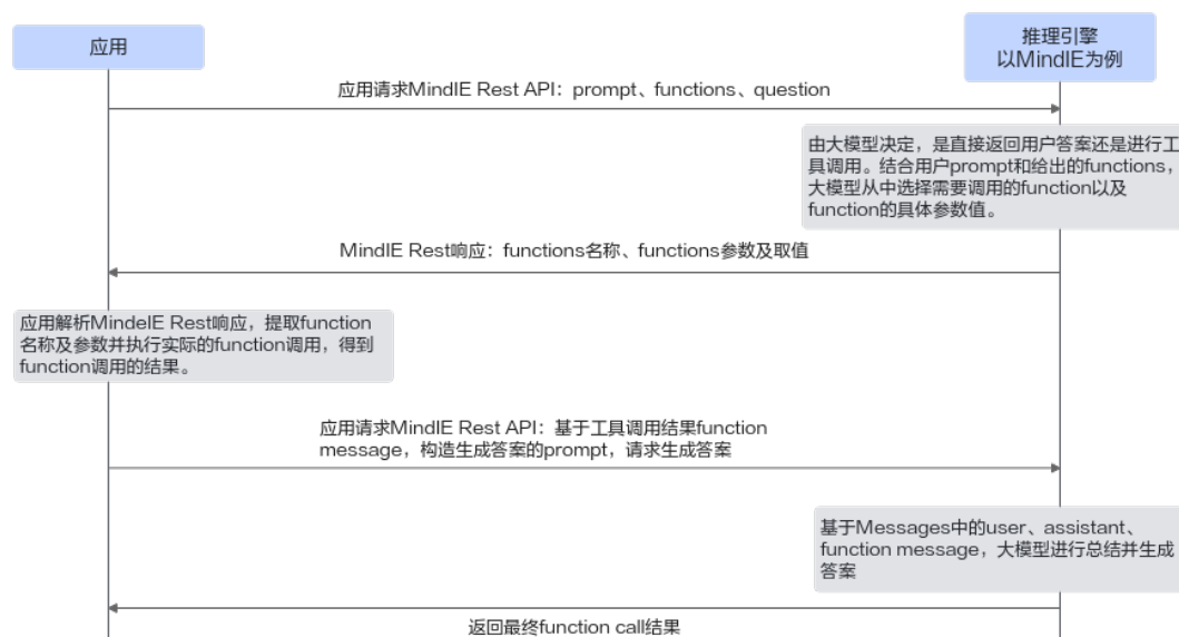
图 7-1 大模型工具调用的流程图
