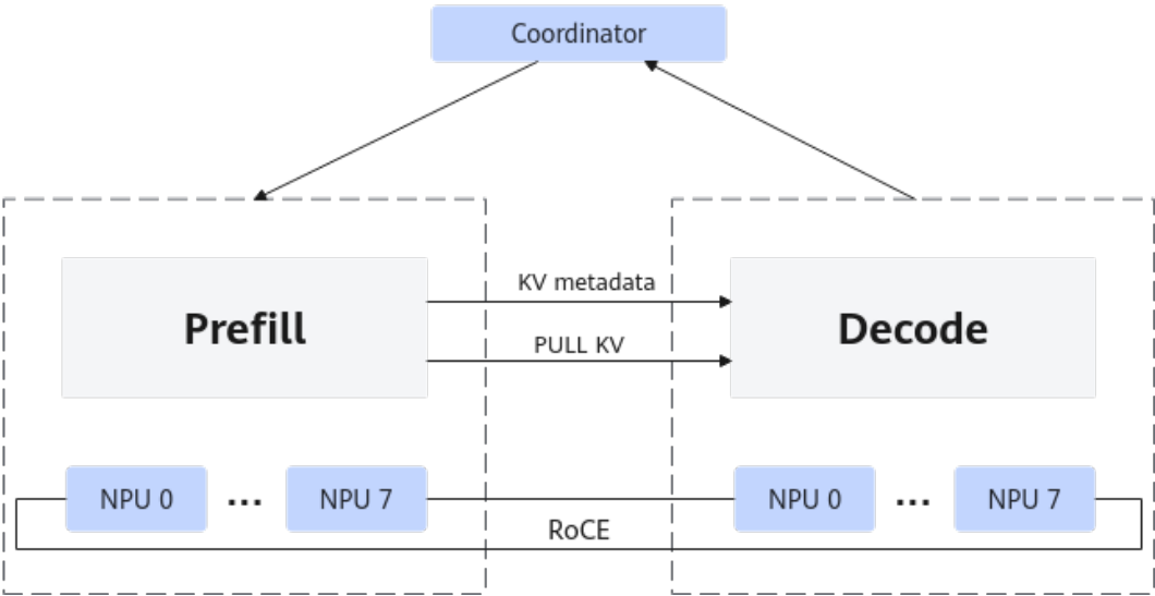
图 3-15 PD 分离工作原理
