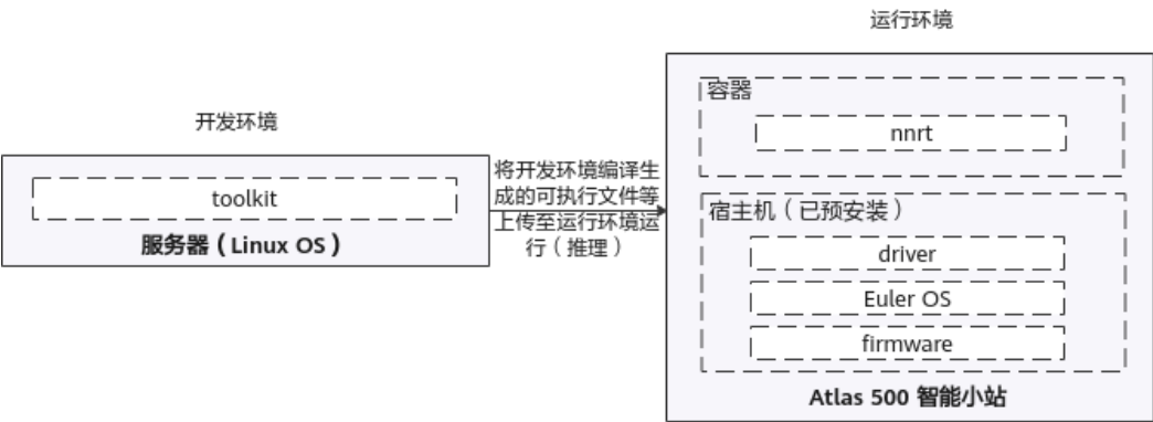
图 2-12 Atlas 500 智能小站
